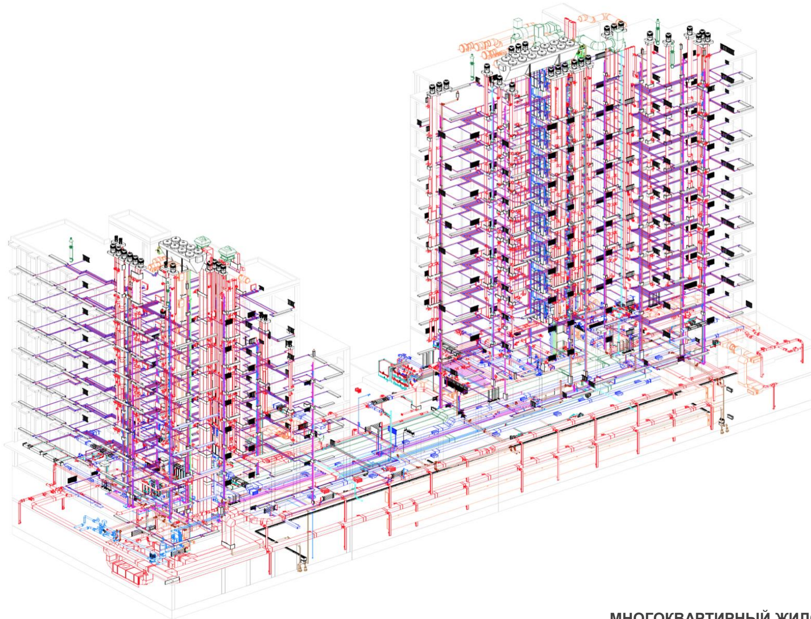
МНОГОВАРТИРНЫЙ ЖИЛОЙ ДОМ Г. МОСКВА СВОДНАЯ МОДЕЛЬ ИНЖЕНЕРНЫХ СЕТЕЙ
